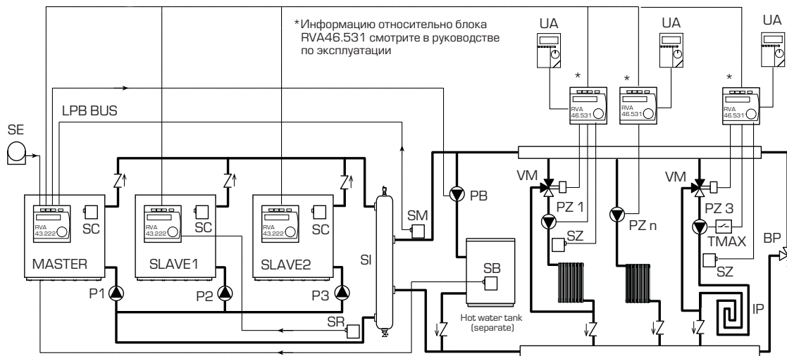
Гидравлическая схема
