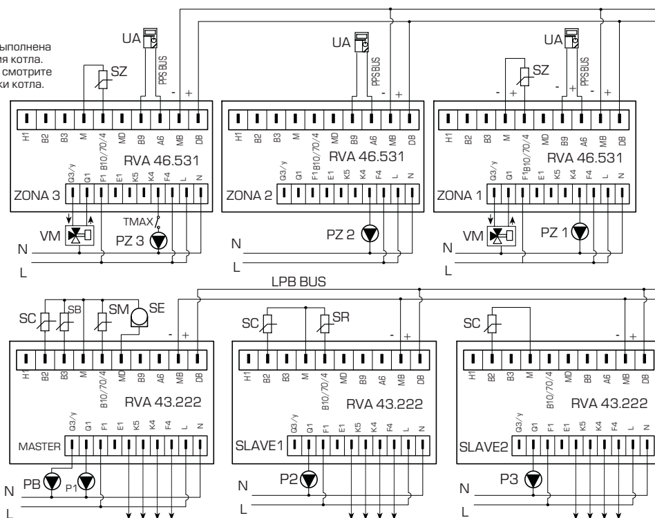
Электрическая схема
